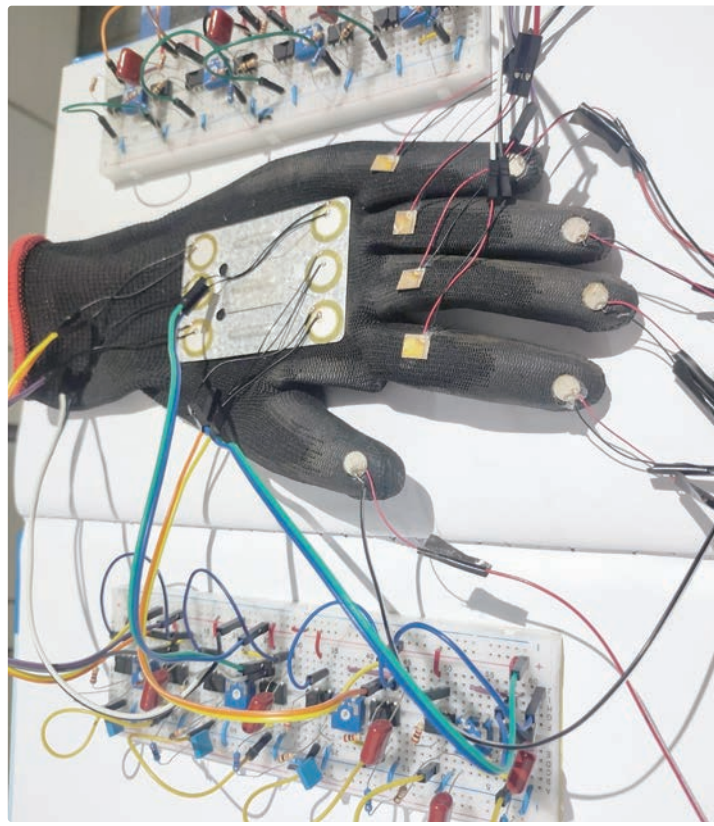
Protótipo vestível instrumentado com sensores e circuitos eletrônicos
